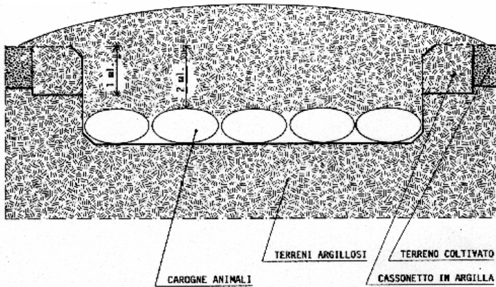
Schema tipo di fossa per la distruzione di carcasse animali di suini affetti da afta epizootica senza raccolta di percolati
