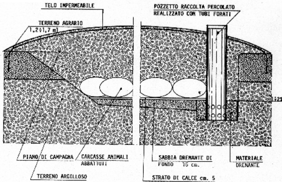
Sezione tipo trasversale
